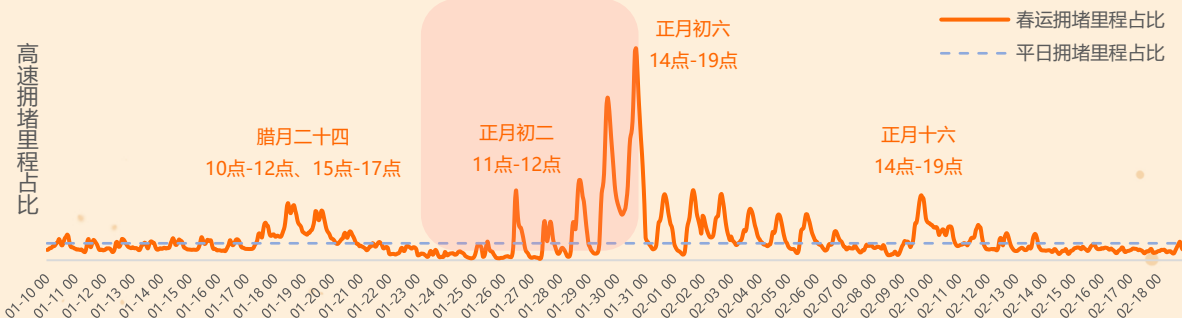
2020年春运期间全国高速公路网拥堵趋势（小时级）
